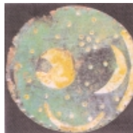
Ο αρχαιότερος αστρικός χάρτης του κόσμου. Ορειχάλκινος δίσκος του 1600 π.Χ. που απεικονίζει τον ουράνιο θόλο με τον Ήλιο, τη Σελήνη και κάποια άστρα φτιαγμένα από χρυσό. Βρέθηκε το 2002 κοντά στην πόλη Nebra της Γερμανίας.
